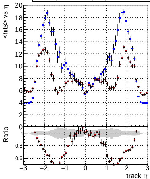
mean hit — DQM_CKF_softQCD — DQM_mkFit_SoftQCD-updated — DQM_mkFit_SoftQCD-updated-newPLDNN
