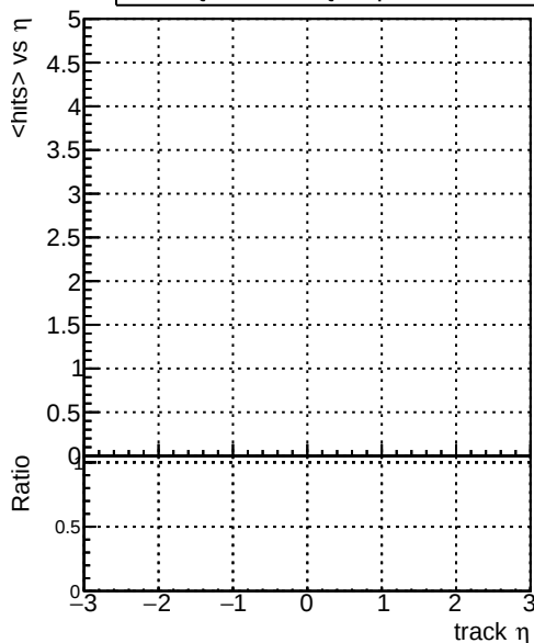
mean hits DQM_CKF_softQCD DQM_mkFit_SoftQCD-updated DQM_mkFit_SoftQCD-updated-newPLDNN
