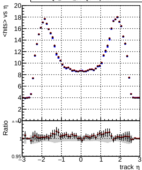
mean hit DQM_CKF_softQCD DQM_mkFit_SoftQCD-updated DQM_mkFit_SoftQCD-updated-newPLDNN
