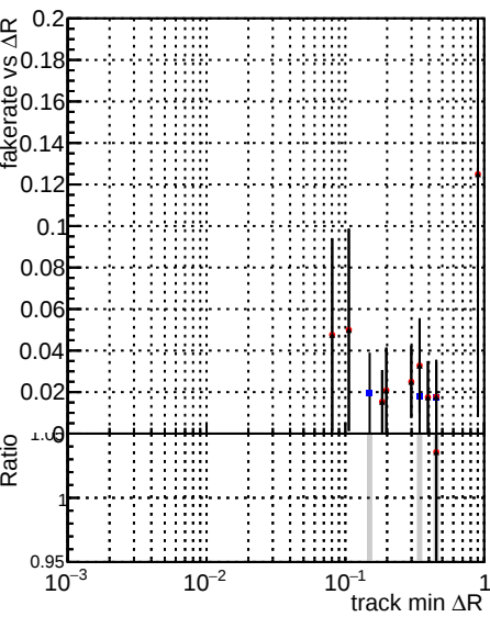
DOM_CKF_softQCD DOM_mkFit_SoftQCD-updated DOM_mkFit_SoftQCD-updated-newPLDNN
