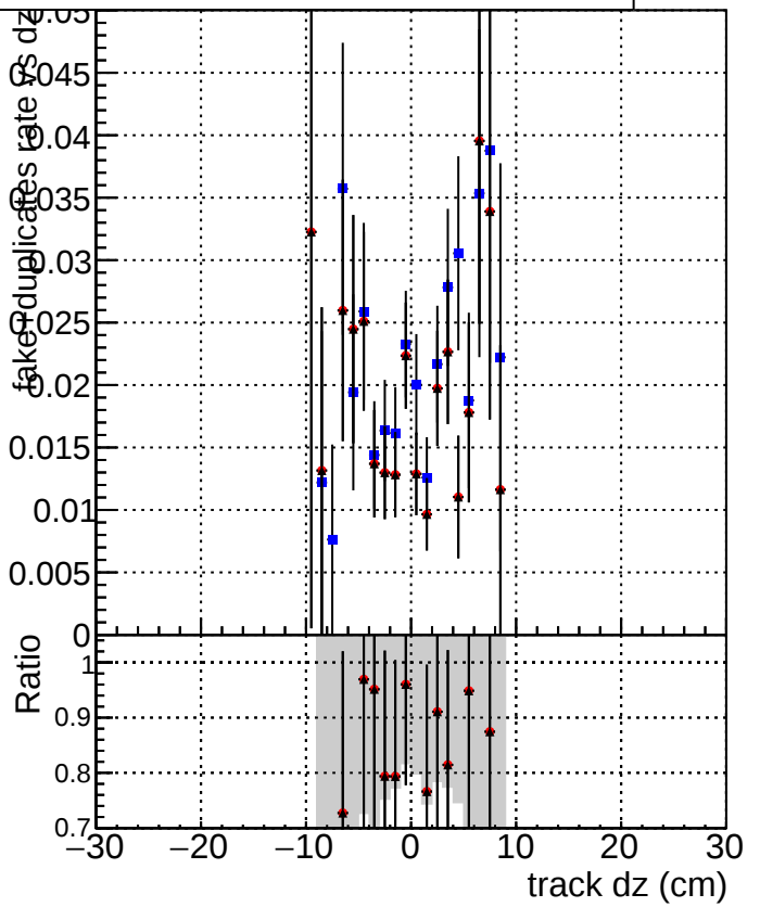
Legend: DQM_CKF_softQCD DQM_mkFit_SoftQCD-updated DQM_mkFit_SoftQCD-updated-newPLDNN
