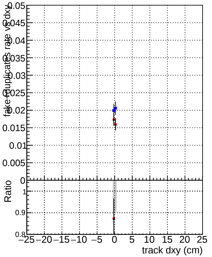
Legend: DQM_CKF_softQCD DQM_mkFit_SoftQCD-updated DQM_mkFit_SoftQCD-updated-newPLDNN
