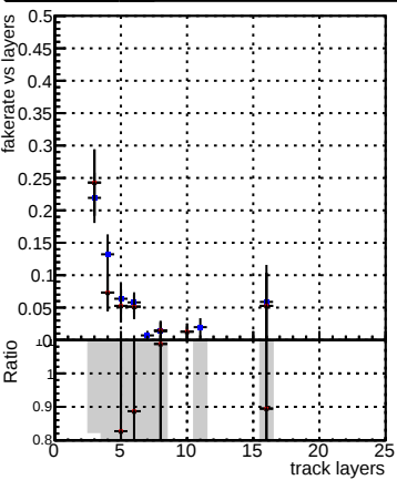
Legend: DQM_CKF_softQCD, DQM_mkFit_SoftQCD-updated, DQM_mkFit_SoftQCD-updated-newPLDNN
