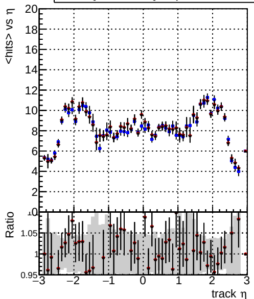
mean hits — DQM_CKF_softQCD — DQM_mkFit_SoftQCD-updated — DQM_mkFit_SoftQCD-updated-newPLDNN
