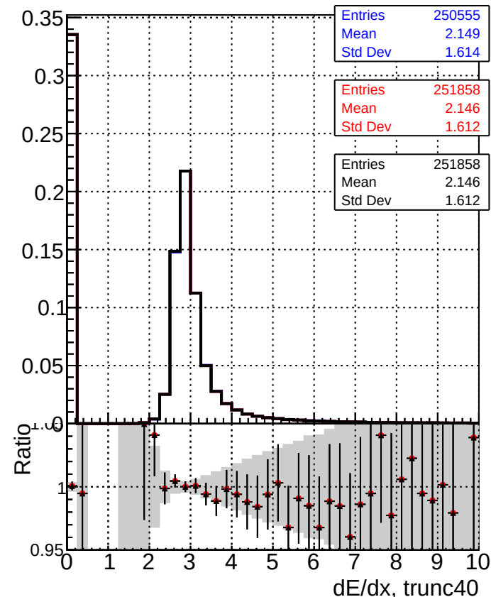
dE/dx estimator 2
