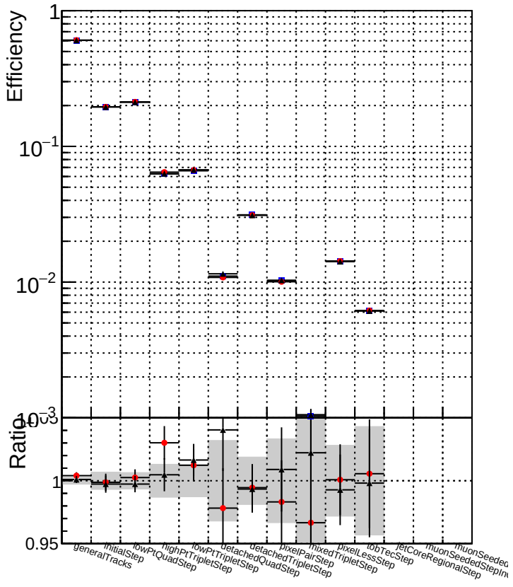
DQM_CKF_TTbase DQM_CKF_TT_retrainOldFiles113 DQM_CKF_TT_retrainOldFiles125_v2
