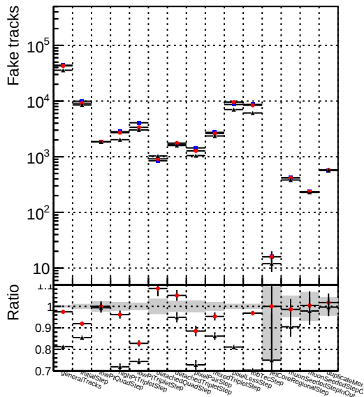
Number ● DQM_CKF_TT_retrainOldFiles113 ★ DQM_CKF_TT_retrainOldFiles125_v2
