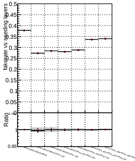
Fake rate vs. DOM CKF TTbase DOM CKF TT retrainOldFiles113 DOM CKF TT retrainOldFiles125 v2
