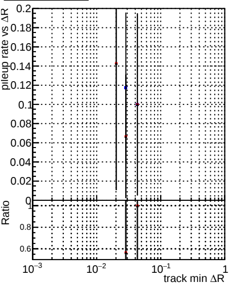
Legend: DQM_CKF_TTbase (grey), DQM_CKF_TT_retrainOldFiles113 (red), DQM_CKF_TT_retrainOldFiles125_v2 (blue)
