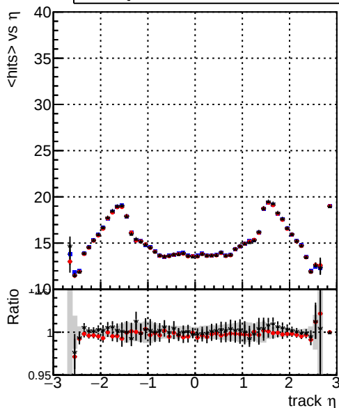
mean hits vs \eta — DQM_CKF_TTbase — DQM_CKF_TT_retrainOldFiles113 — DQM_CKF_TT_retrainOldFiles125_v2
