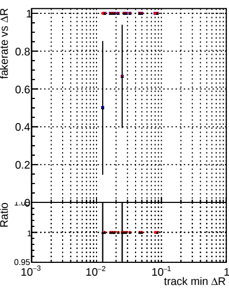
Fake rate vs \Delta R(\text{track, jet}) DQM_CKF_TTbase DQM_CKF_TT_retrainOldFiles113 DQM_CKF_TT_retrainOldFiles125_v2
