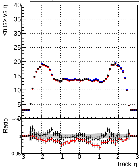
mean hits > \eta — DQM_CKF_TTbase — DQM_CKF_TT_retrainOldFiles113 — DQM_CKF_TT_retrainOldFiles125_v2
