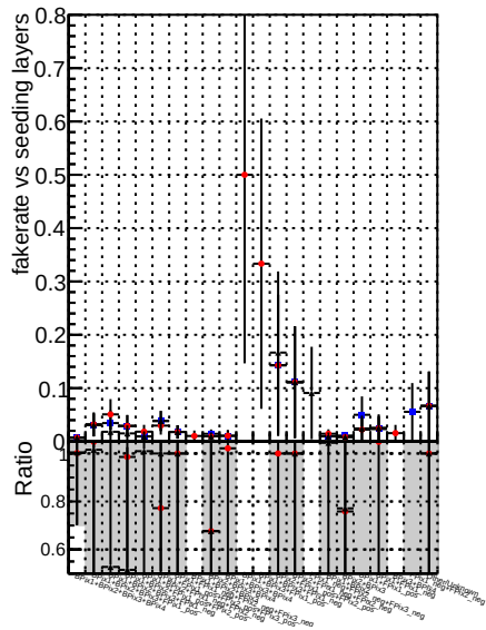
Fake rate vs. DOM CKF TTbase DOM CKF TTbase retrainOldFiles113 DOM CKF TTbase retrainOldFiles125 v2
