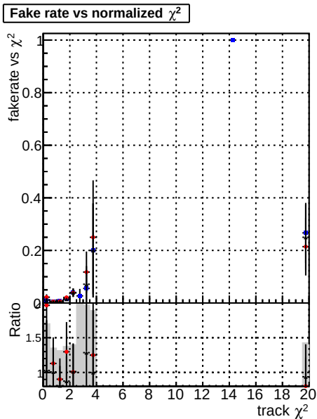
Fake rate vs. DOM CKF TTbase DOM CKF TTbase retrainOldFiles113 DOM CKF TTbase retrainOldFiles125 v2
