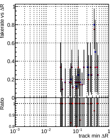
DOM_CKF_TTbase DOM_CKF_TT_retrainOldFiles113 DOM_CKF_TT_retrainOldFiles125_v2
