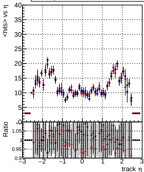
mean hits — DQM_CKF_TTbase — DQM_CKF_TT_retrainOldFiles113 — DQM_CKF_TT_retrainOldFiles125_v2
