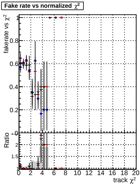
Fake rate vs. DOM CKF TTbase DOM CKF retrainOldFiles113 DOM CKF retrainOldFiles125 v2
