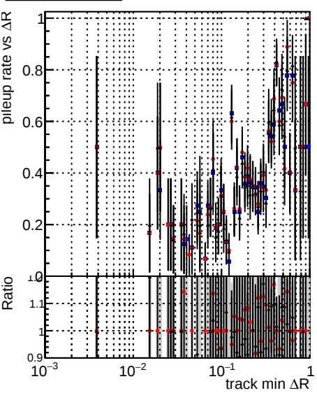
—•— DQM_CKF_TTbase —•— DQM_CKF_TT_retrainOldFiles113 —•— DQM_CKF_TT_retrainOldFiles125_v2
