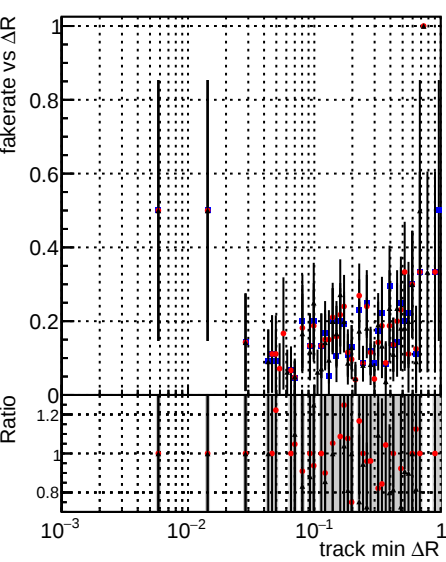
—•— DQM_CKF_TTbase —•— DQM_CKF_TT_retrainOldFiles113 —•— DQM_CKF_TT_retrainOldFiles125_v2
