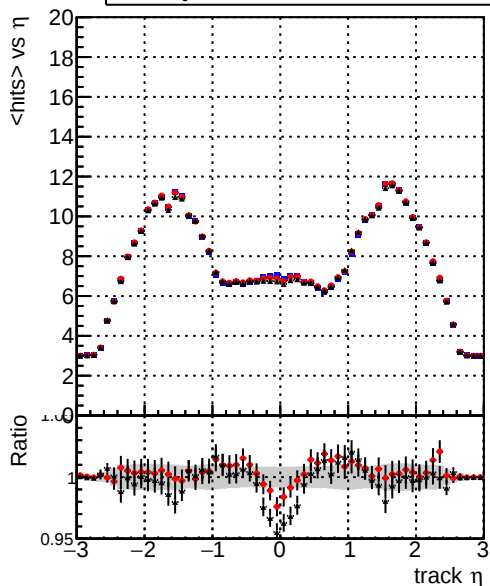
mean hits vs \eta — DQM_CKF_TTbase — DQM_CKF_TT_retrainOldFiles113 — DQM_CKF_TT_retrainOldFiles125_v2
