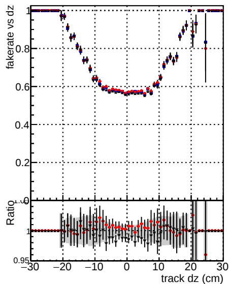
Fake rate vs d DOM CKE TTbase DOM CKE TT retrainOldFiles113 DOM CKE TT retrainOldFiles125 v2
