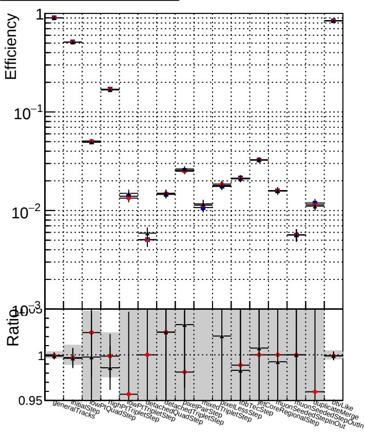
DQM_CKF_TTbase DQM_CKF_TT_retrainOldFiles113 DQM_CKF_TT_retrainOldFiles125_v2
