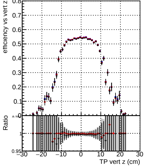
Efficiency vs. sim PV z —●— DQM_CKF_TTbase —●— DQM_CKF_TT_retrainOldFiles113 —●— DQM_CKF_TT_retrainOldFiles125_v2
