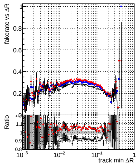
DOM_CKF_TTbase DOM_CKF_TT_retrainOldFiles113 DOM_CKF_TT_retrainOldFiles125_v2
