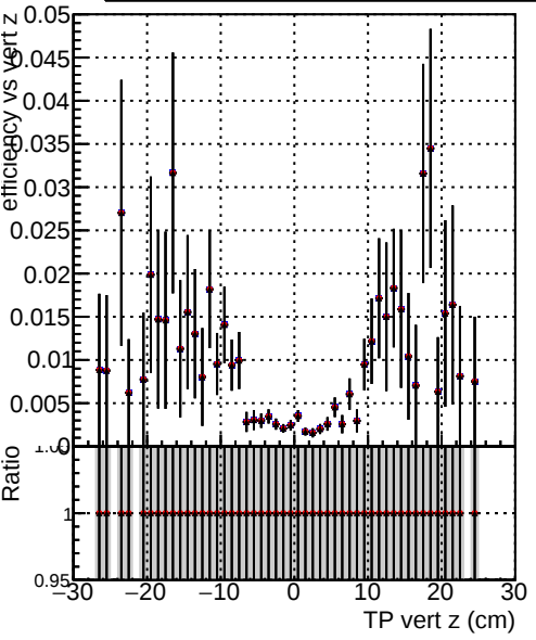
Efficiency vs TP vert z (cm) Legend: DQM_CKF_TT_base_noSel DQM_CKF_TT_retrainOldFiles113_noSel DQM_CKF_TT_retrainOldFiles125_v2_noSel
