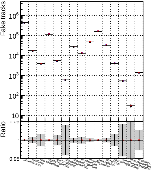
Number File 1 DQM_CKF_TT_retrainOldFiles113_noSel 2 DQM_CKF_TT_retrainOldFiles125_v2_noSel
