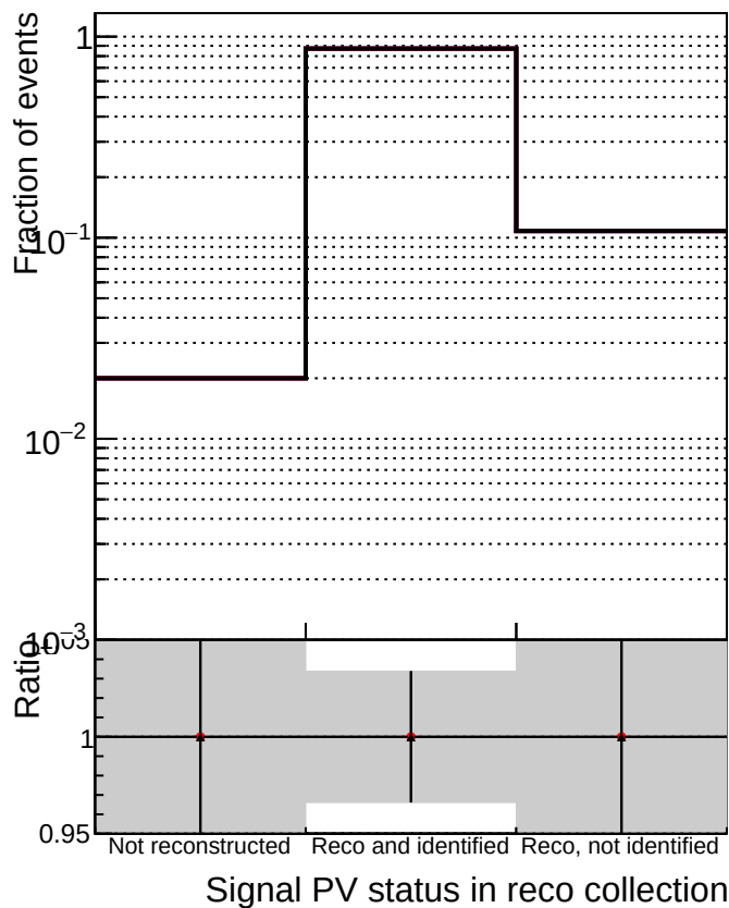
—■ DQM_CKF_TT_base_noSel —● DQM_CKF_TT_retrainOldFiles113_noSel —▲ DQM_CKF_TT_retrainOldFiles125_v2_noSel
