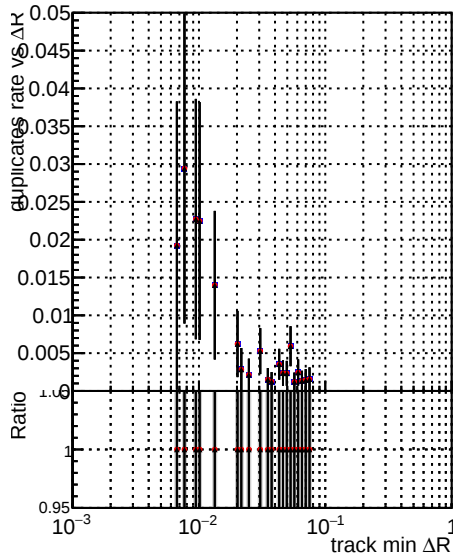
—•— DQM_CKF_TT_base_noSel —•— DQM_CKF_TT_retrainOldFiles113_noSel —•— DQM_CKF_TT_retrainOldFiles125_v2_noSel
