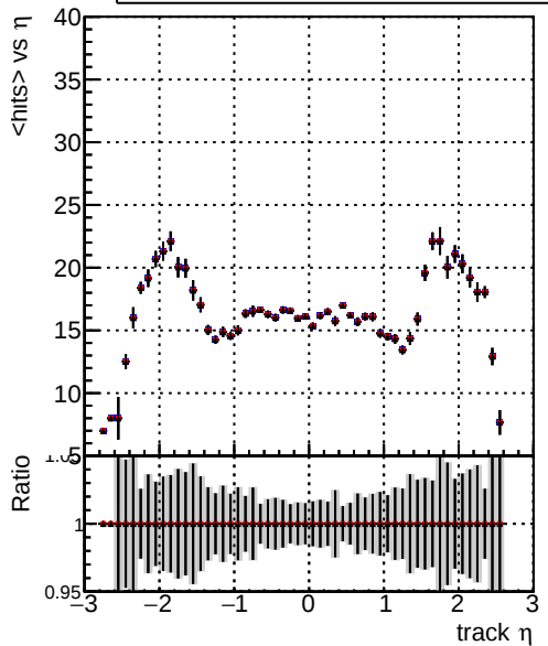
mean hits vs \eta — DQM_CKF_TT_base_noSel — DQM_CKF_TT_retrainOldFiles113_noSel — DQM_CKF_TT_retrainOldFiles125_v2_noSel
