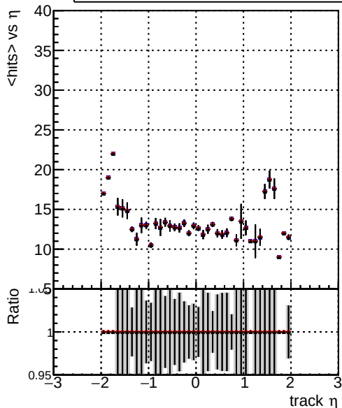
mean hits DQM_CKF_TT_base_noSel DQM_CKF_TT_retrainOldFiles113_noSel DQM_CKF_TT_retrainOldFiles125_v2_noSel
