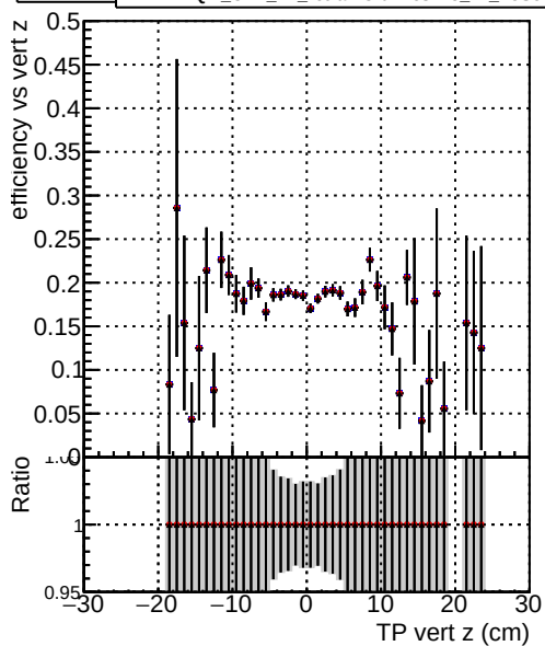
—●— DQM_CKF_TT_base_noSel —●— DQM_CKF_TT_retrainOldFiles113_noSel —●— DQM_CKF_TT_retrainOldFiles125_v2_noSel
