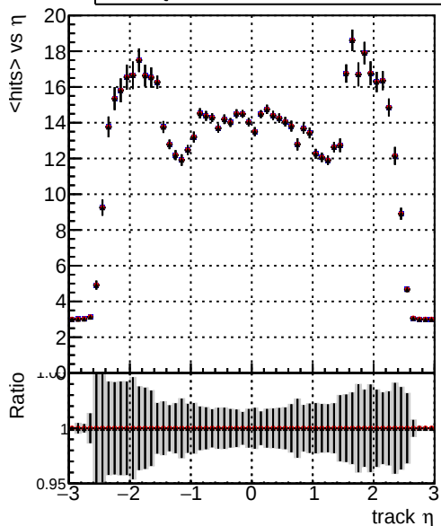
mean hit — DQM_CKF_TT_base_noSel — DQM_CKF_TT_retrainOldFiles113_noSel — DQM_CKF_TT_retrainOldFiles125_v2_noSel
