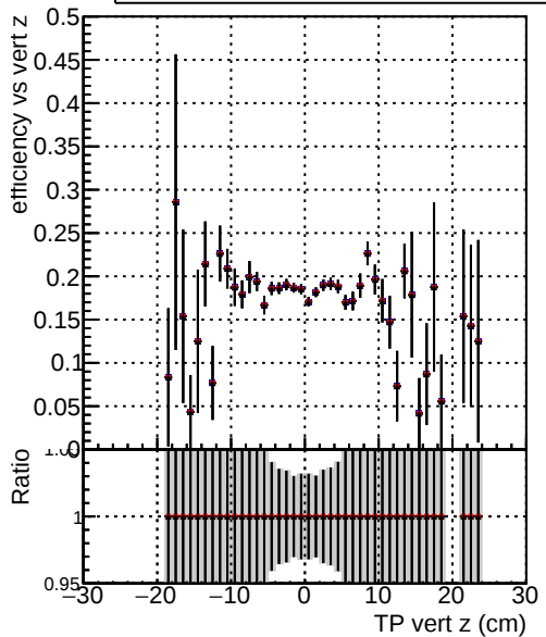
Efficiency vs. sim PV z — DQM_CKF_TT_base_noSel — DQM_CKF_TT_retrainOldFiles113_noSel — DQM_CKF_TT_retrainOldFiles125_v2_noSel
