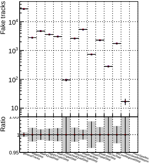
Number Model 1 DQM_CKF_TT_retrainOldFiles113_noSel 2 DQM_CKF_TT_retrainOldFiles125_v2_noSel
