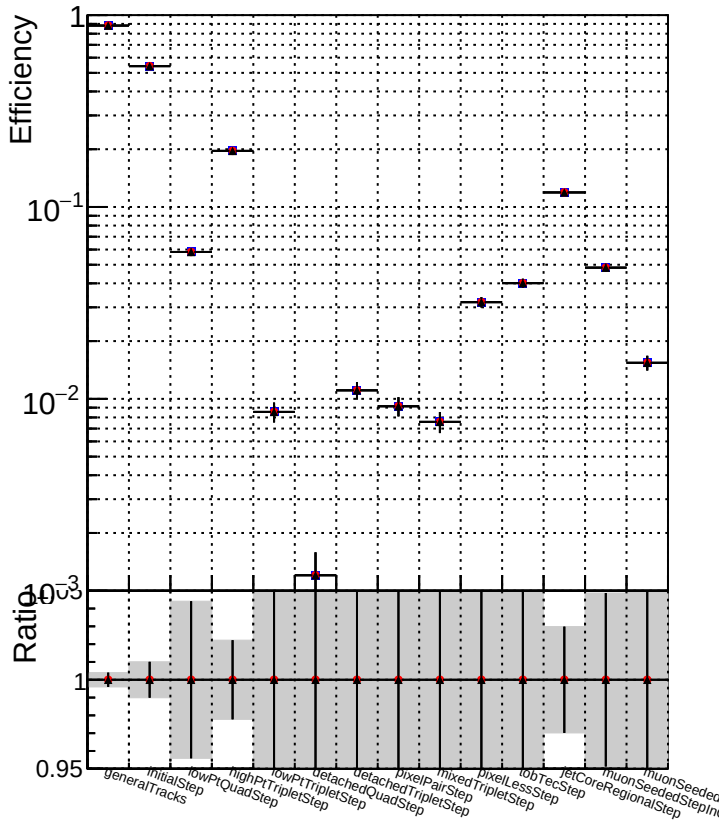
DQM_CKF_TT_base_noSel DQM_CKF_TT_retrainOldFiles113_noSel DQM_CKF_TT_retrainOldFiles125_v2_noSel
