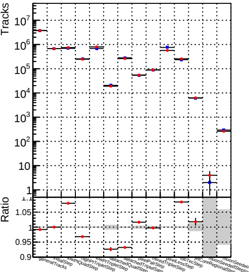
■ DQM_mkFit_TT_base_noSel
