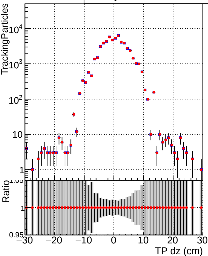
■ DQM_mkFit_TT_base_noSel ■ DQM_mkFit_TT_retrainOldFiles_v2_8iter_noSel
