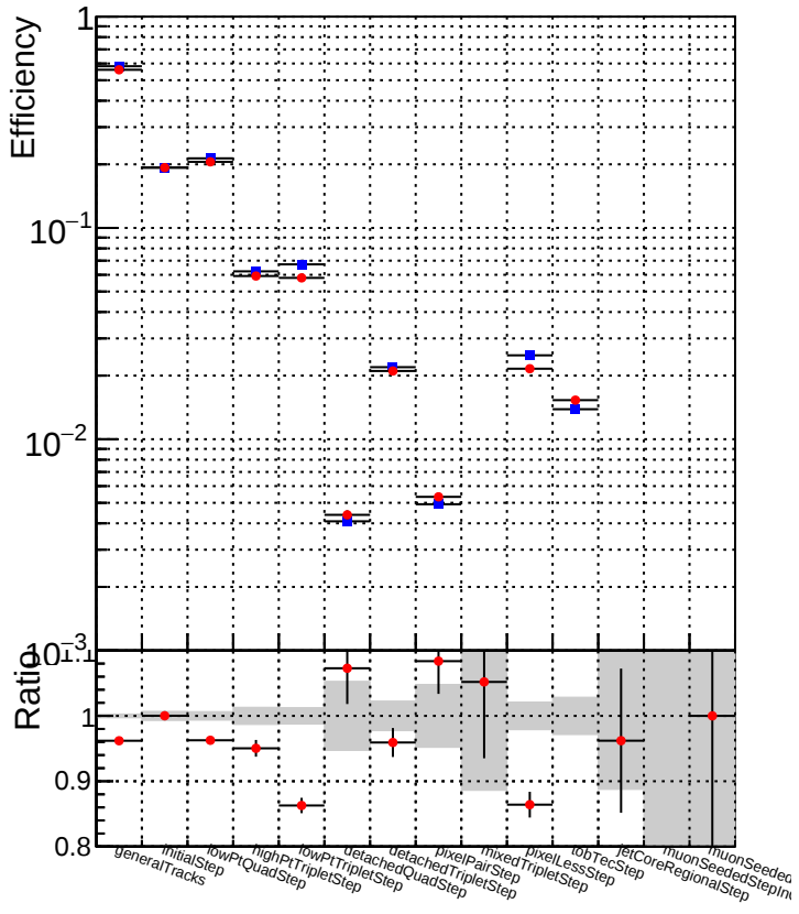
DQM_mkFit_TT_base_noSel DQM_mkFit_TT_retrainOldFiles_v2_8iter2_noSel
