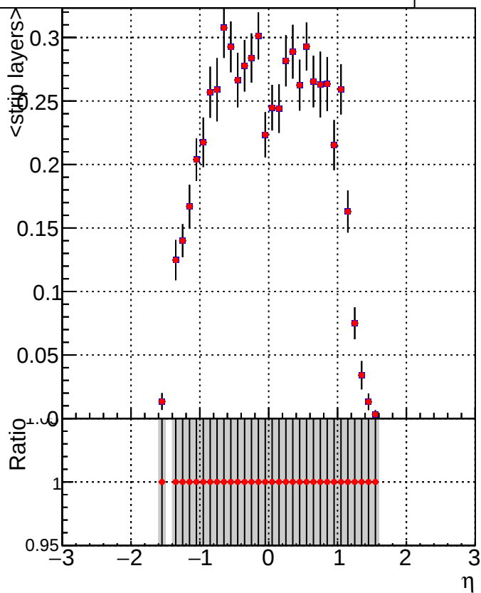
DQM_mkFit_TT_base_noSel DQM_mkFit_TT_retrainOldFiles_v2_8iter2_noSel
