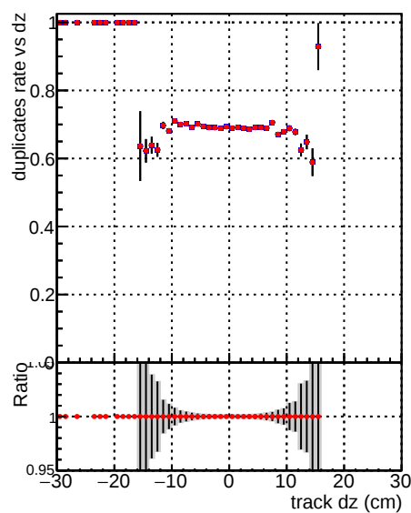
— DQM_mkFit_TT_base_noSel — DQM_mkFit_TT_retrainOldFiles_v2_8iter2_noSel
