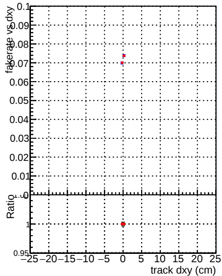
— DQM_mkFit_TT_base_noSel — DQM_mkFit_TT_retrainOldFiles_v2_8iter2_noSel
