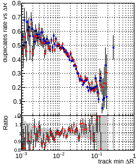
— \Delta R DQM_mkFit_TT_base_noSel — \Delta R DQM_mkFit_TT_retrainOldFiles_v2_8iter2_noSel
