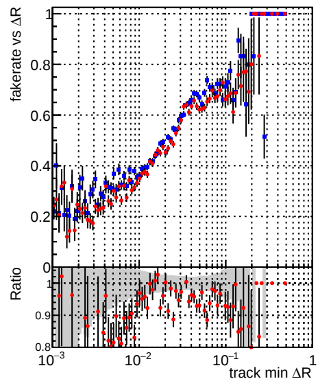
— \Delta R DQM_mkFit_TT_base_noSel — \Delta R DQM_mkFit_TT_retrainOldFiles_v2_8iter2_noSel
