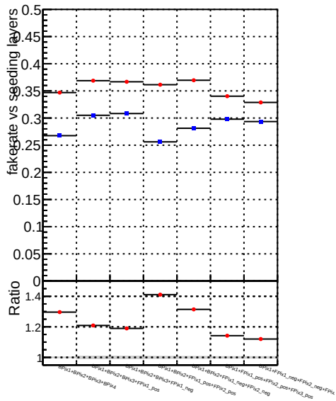
Fake rate vs. DQM mkFit TT base_noSel DQM mkFit TT retrainOldFiles_v2 8iter2_noSel
