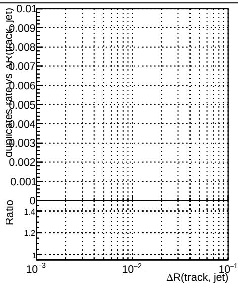
—•— DQM_mkFit_TT_base_noSel —•— DQM_mkFit_TT_retrainOldFiles_v2_8iter2_noSel
