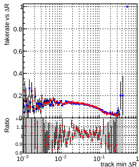
—•— DQM_mkFit_TT_base_noSel —•— DQM_mkFit_TT_retrainOldFiles_v2_8iter2_noSel
