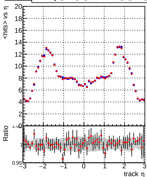
— DQM_mkFit_TT_base_noSel — DQM_mkFit_TT_retrainOldFiles_v2_8iter2_noSel
