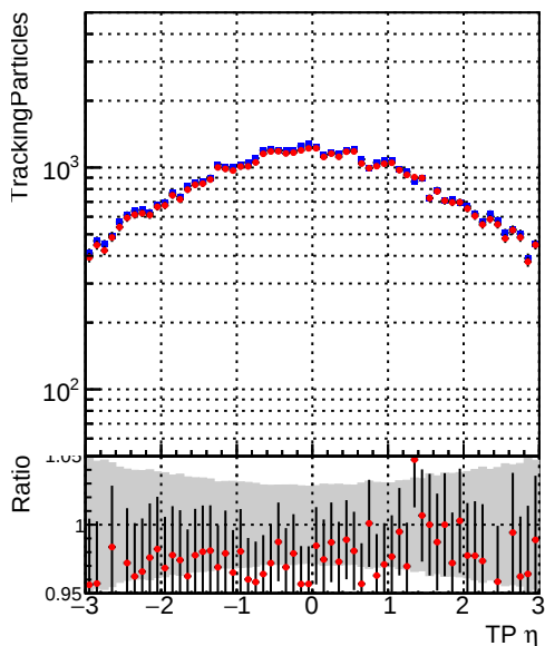
—•— DQM_mkFit_TT_base_noSel —•— DQM_mkFit_TT_retrainOldFiles_v2_8iter2_noSel
