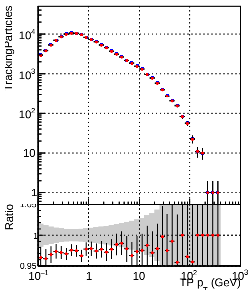
—•— DQM_mkFit_TT_base_noSel —•— DQM_mkFit_TT_retrainOldFiles_v2_8iter2_noSel
