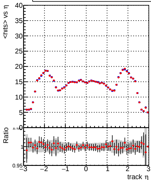
— DQM_mkFit_TT_base_noSel — DQM_mkFit_TT_retrainOldFiles_v2_8iter2_noSel mean hits
