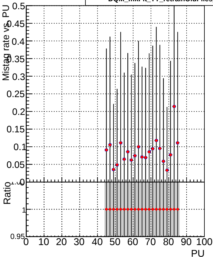
■ DQM_mkFit_TT_base_noSel ● DQM_mkFit_TT_retrainOldFiles_v2_8iter2_noSel
