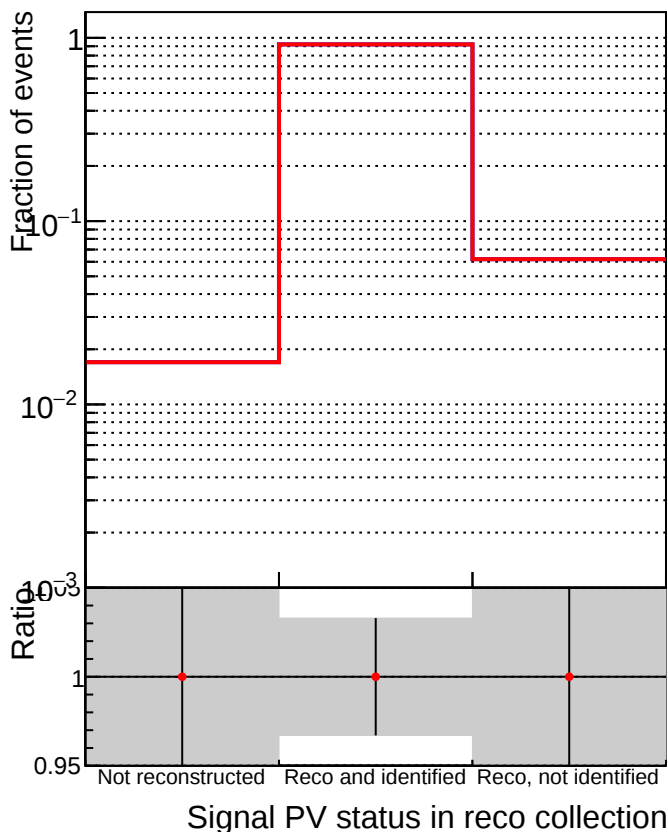
■ DQM_mkFit_TT_base_noSel ● DQM_mkFit_TT_retrainOldFiles_v2_8iter2_noSel
