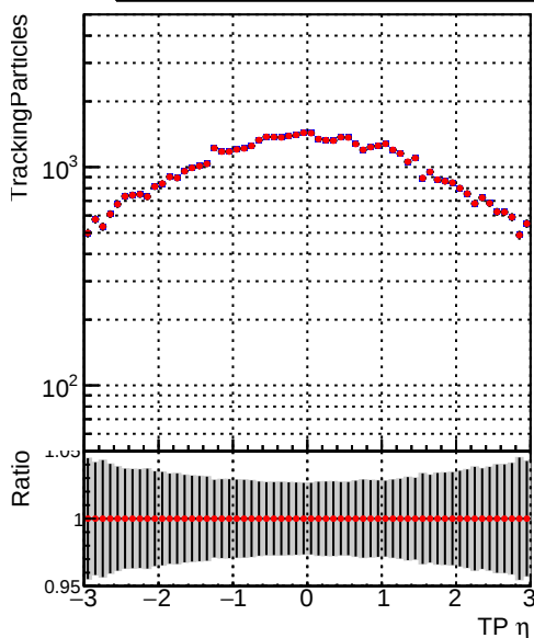
—•— DQM_mkFit_TT_base_noSel —•— DQM_mkFit_TT_retrainOldFiles_v2_8iter2_noSel
