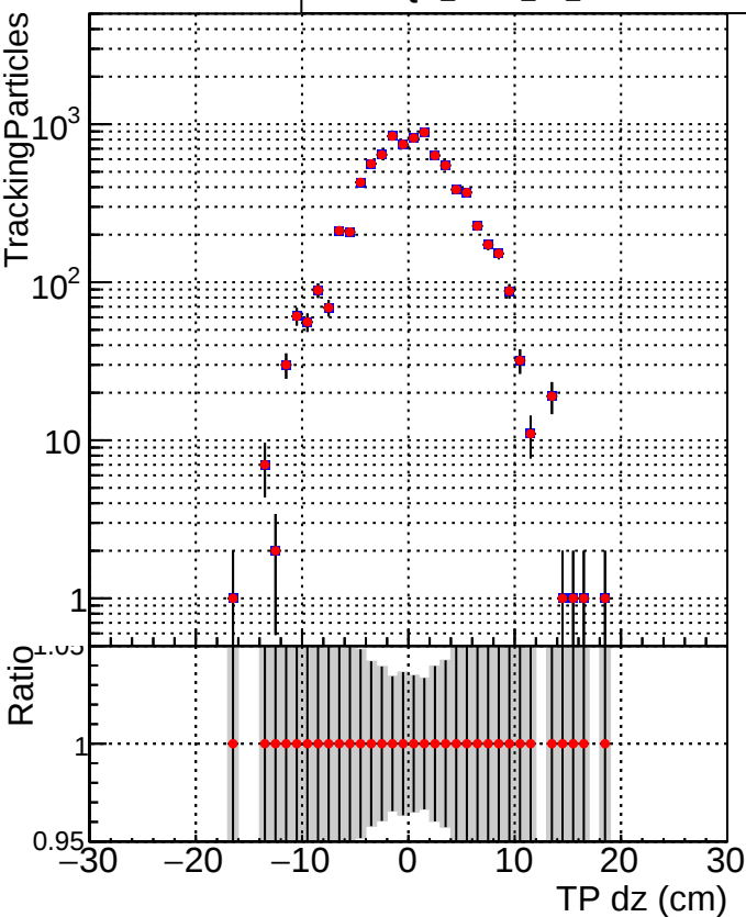
■ DQM_mkFit_TT_base_noSel ■ DQM_mkFit_TT_retrainOldFiles_v2_8iter2_noSel
