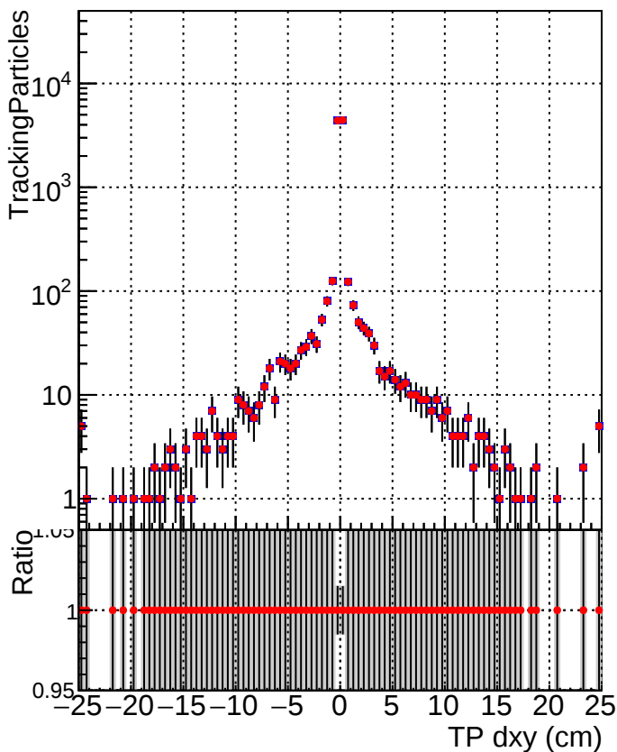
■ DQM_mkFit_TT_base_noSel ■ DQM_mkFit_TT_retrainOldFiles_v2_8iter2_noSel
